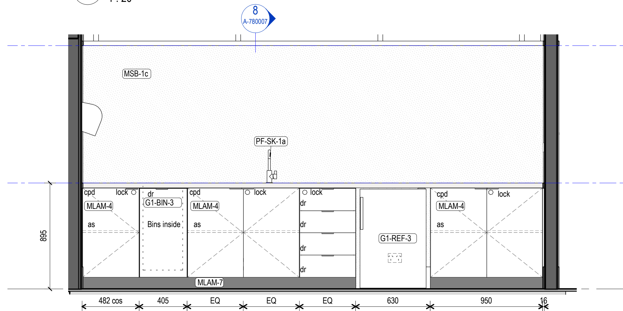
7 JO-BW-6 Elevation 1 : 20
