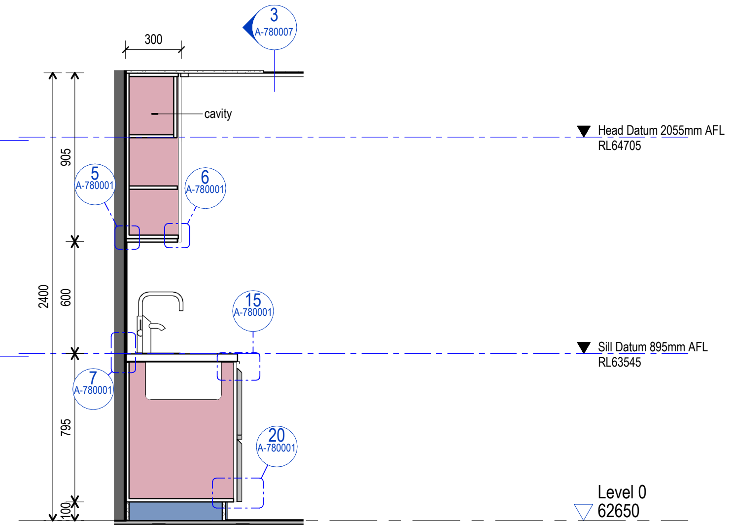
4 JO-BW-5 Section 1 : 20
