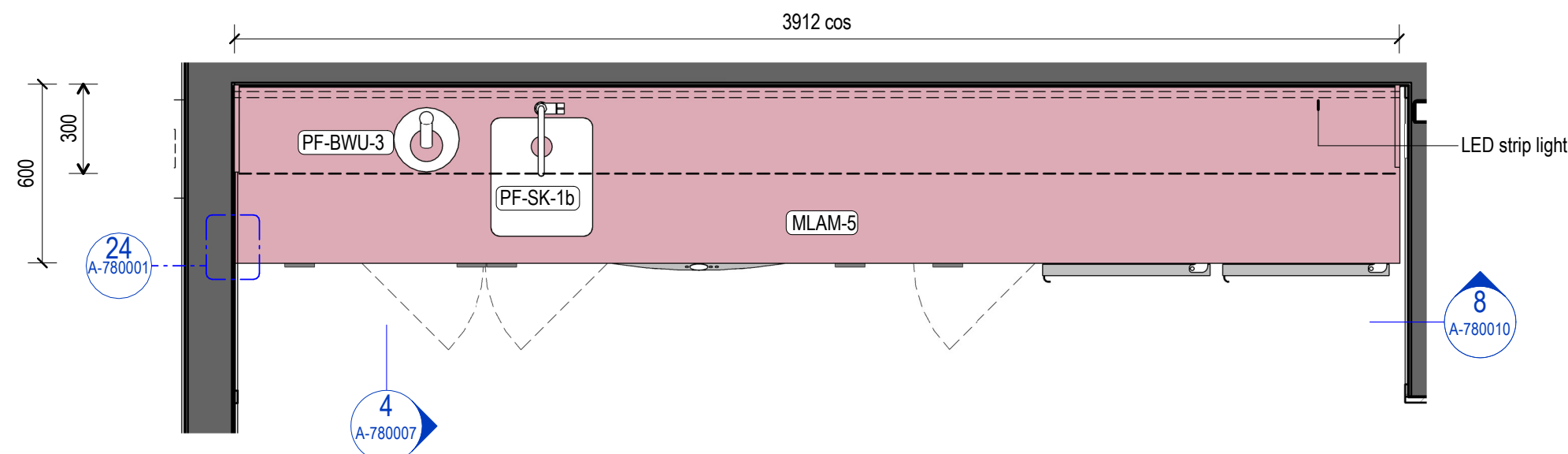
2 JO-BW-5 - Plan 1 : 20
