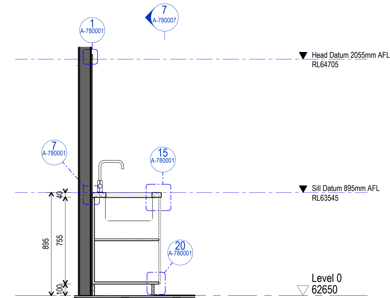
8 JO-BW-6 Section 1 : 20
