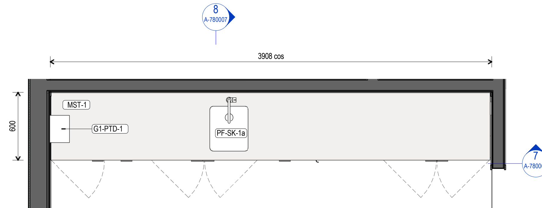
6 JO-BW-6 Plan 1 : 20
